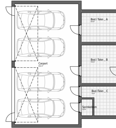
Plan Kjeller av Bygg A, Bod og garasje plass, Mål 1:200
